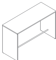
PSW78 1800 / 700 / 1100 64.2 kg
