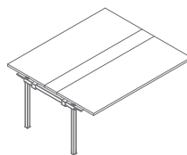
SY36 1600 / 1410 / 740 66.8 kg
