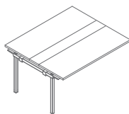
SY54 1400 / 1210 / 740 54.15 kg
