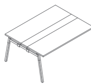
SW26L 1600 / 1210 / 740 57 kg
